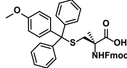
Fmoc-(Me)Cys(Mmt)-OH
