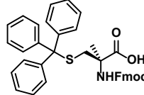
Fmoc-(Me)Cys(Trt)-OH
