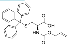
Aloc-Cys(Trt)-OH
