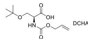
Aloc-Ser(tBu)-OH·DCHA
