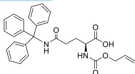
Aloc-Gln(Trt)-OH
