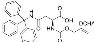
Aloc-Asn(Trt)-OH·DCHA
