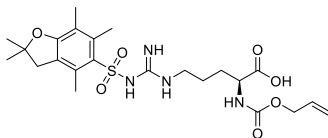
Aloc-Arg(Pbf)-OH
