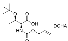
Aloc-Thr(tBu)-OH·DCHA
